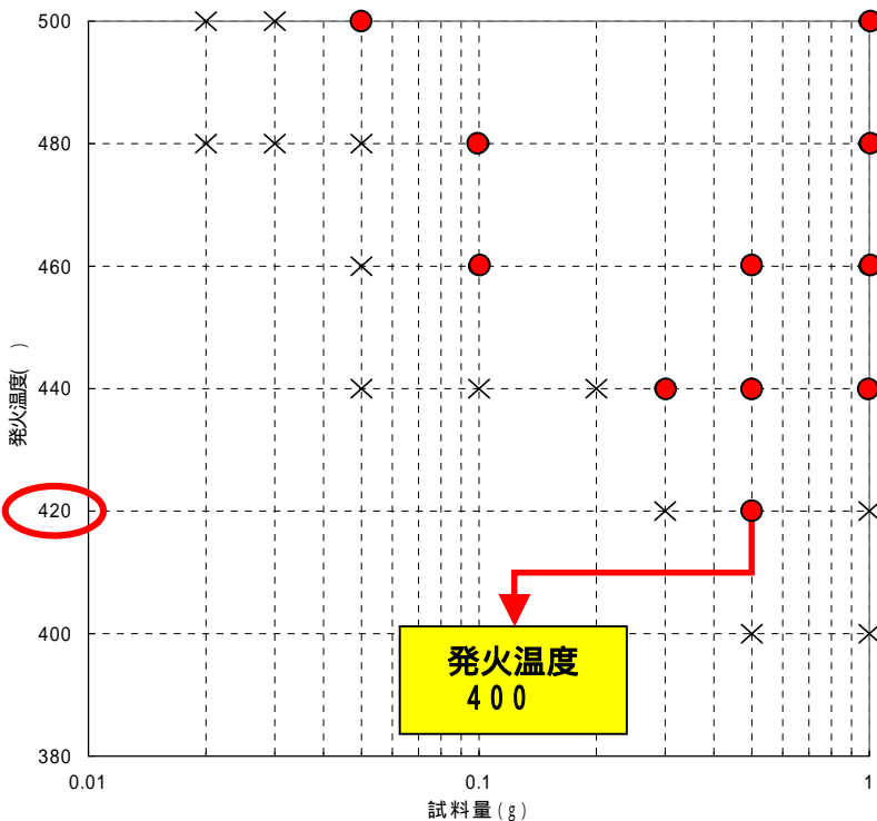
発火温度と試料量の関係
